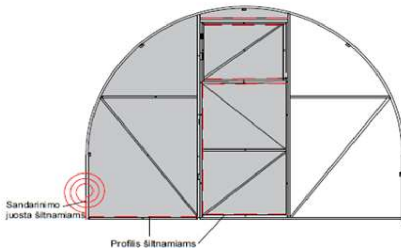
Pav. 18 Polikarbonato dangos montavimas ant šiltnamio rėmo
