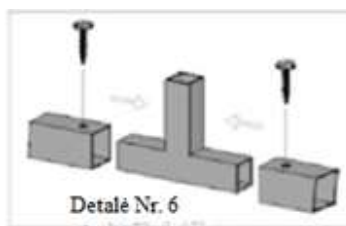
Pav. 9. Savisriegių varžtų tvirtinimo schema
