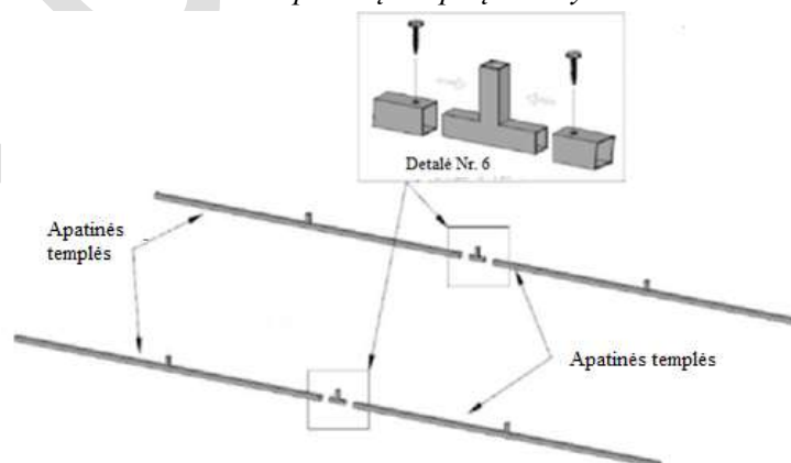
Pav. 7. Apatinių templių išdėstymas
