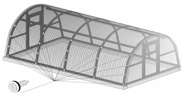
Pav. 16. Savisriegių varžtų tvirtinimo mazgai šiltnamio viršutinėje dalyje
