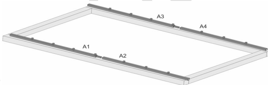
Pav. 7. Apatinių templių išdėstymas
