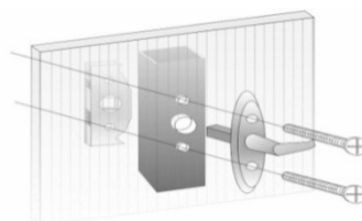
Pav. 5. Durų rankenos įstatymas
