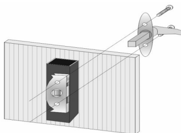
Pav. 6. Durų spynos tvirtinimas
