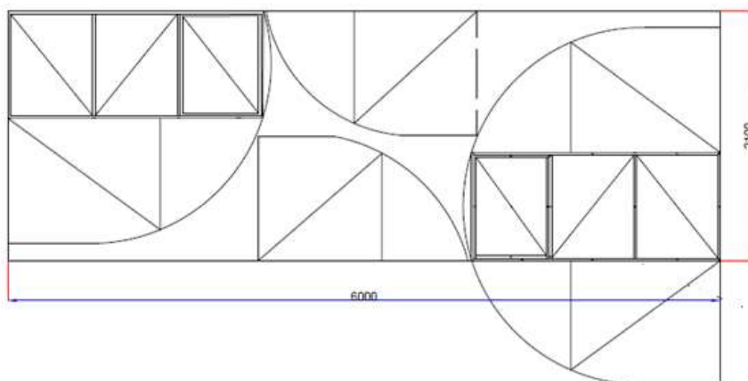
Pav. 2 Polikarbonato pjovimas
